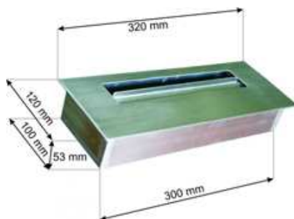
Typy hořáků - nálevek
